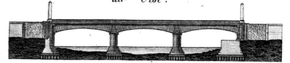
Fig. 48. A. Brücke von Pont-Sainte-Maxence über die Oise.
