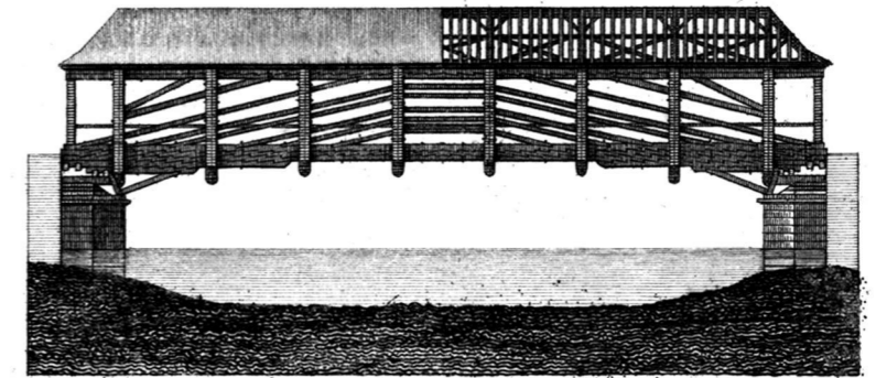
Fig. 10. Brücke von Zürich über die Limmat.
