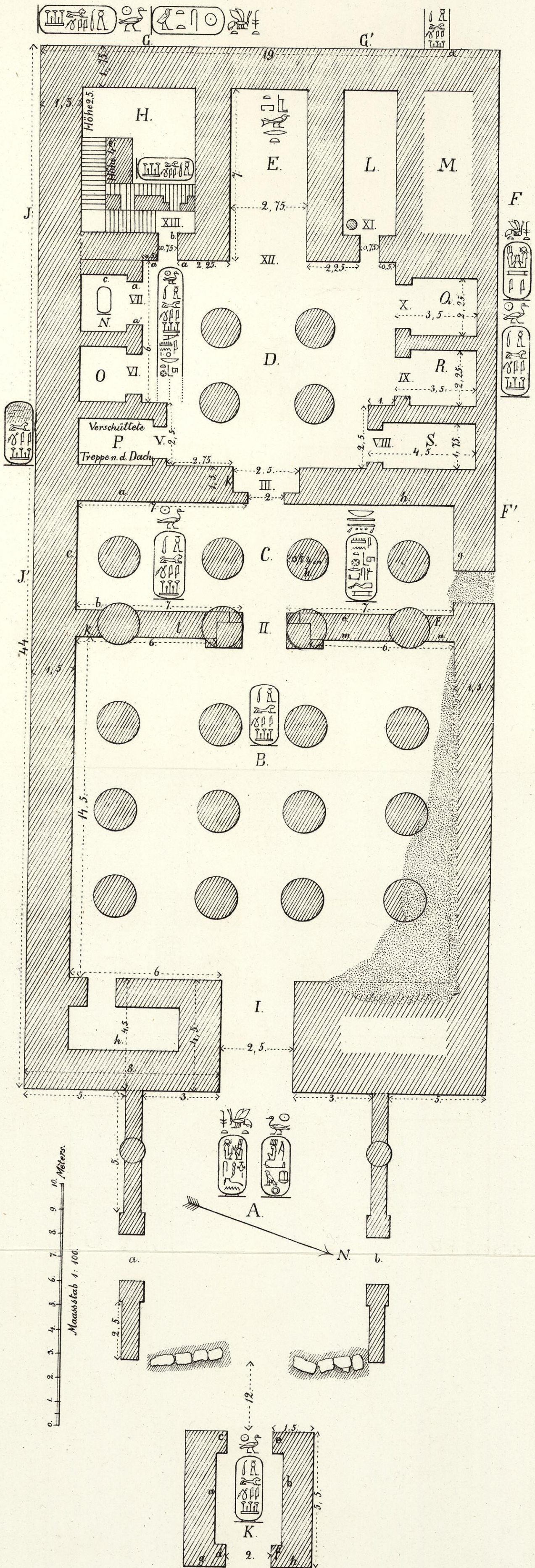
GRUNDPLAN DES TEMPELS VON HIBE.
