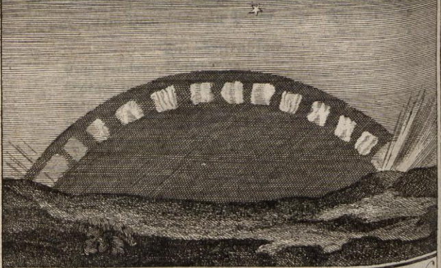
Ein Nordlicht, welches H r . von Mairan 1726. d. 19. Octobr. zu Breuillepont.
