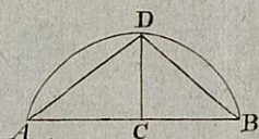
Fig. 29. Prep. XXIX. Fig. 30.
