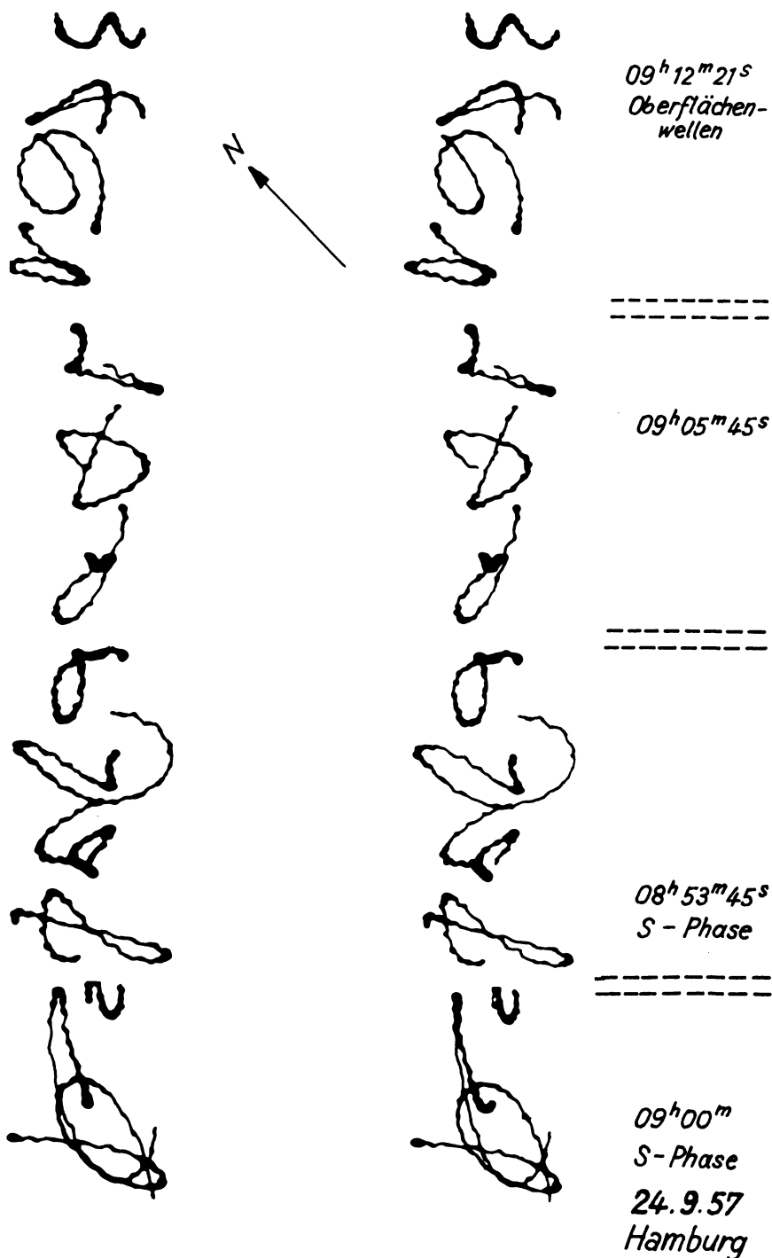
Abb. 4: Ausschnitte aus der stereoskopischen Registrierung eines Erdbebens.
